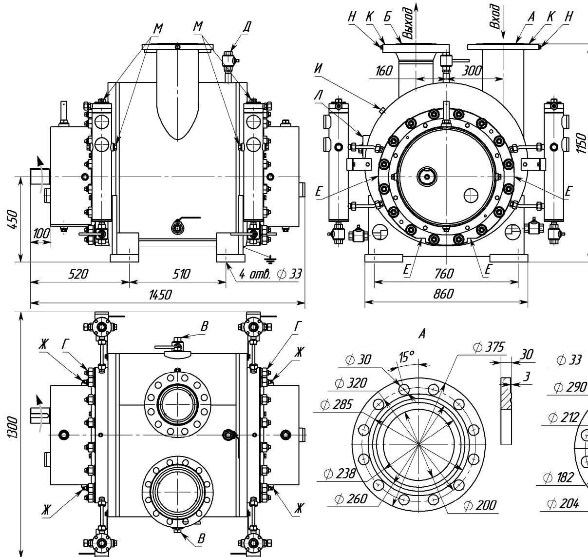
Рисунок Б1 - Габаритный чертеж насоса типа А8 2ВВ140/63, А8 2ВВ200/40
